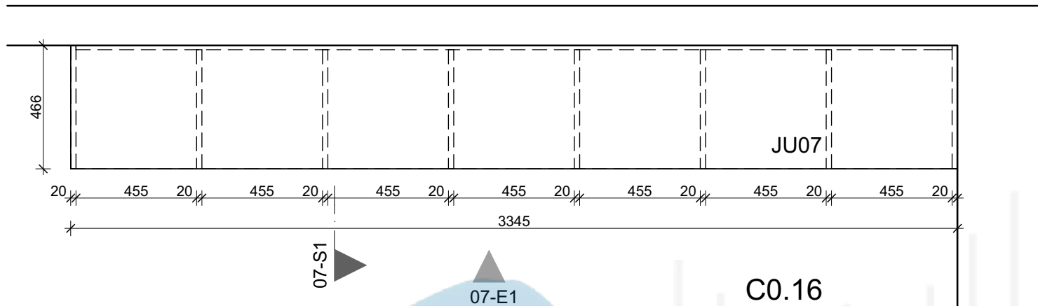
JU07 PLAN 1:20
